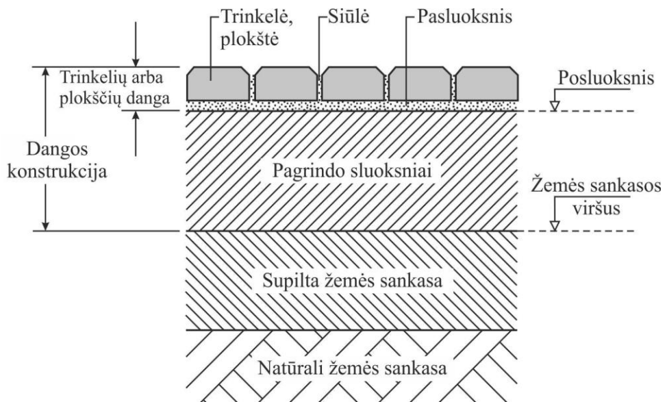
1 pav. Eismo zonos (kelio) konstrukcijos pavidalinė struktūra
